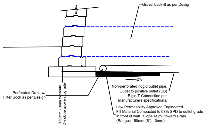
Typ. Section
